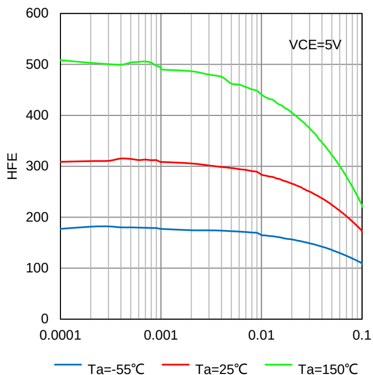
HFE vs. I_C
